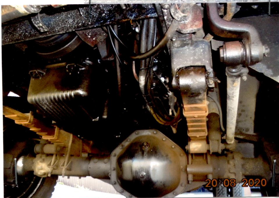
(21) Ujęcie napędu na przednią oś .Widoczne wycieki oleju z silnika na misie olejowej silnika! .
