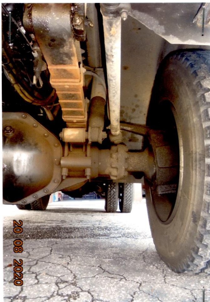
Samochód specjalny pożarniczy JELCZ 244
